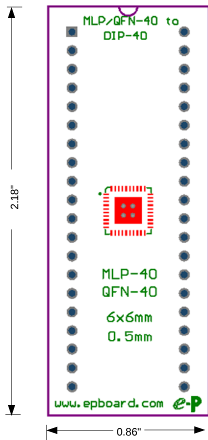
Top Side
