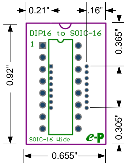
Top Side
